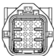
档位执行器连接器
