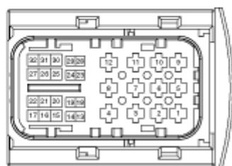
TCM 连接器 [A]
