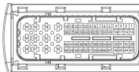
TCM 连接器 [B]
